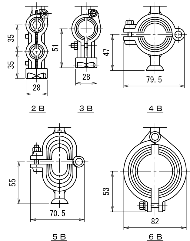
ブラケット
